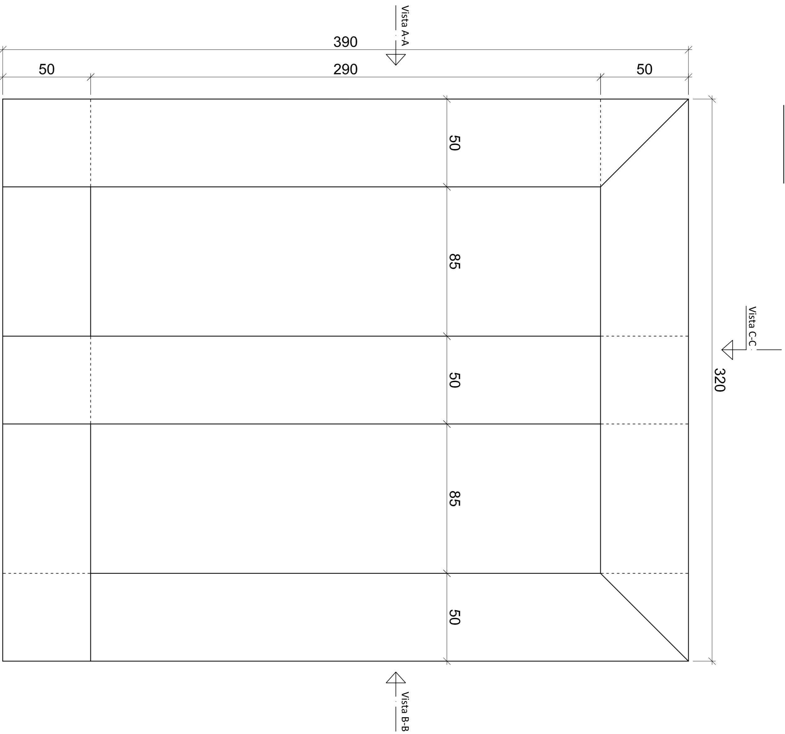
Vista Frontale
