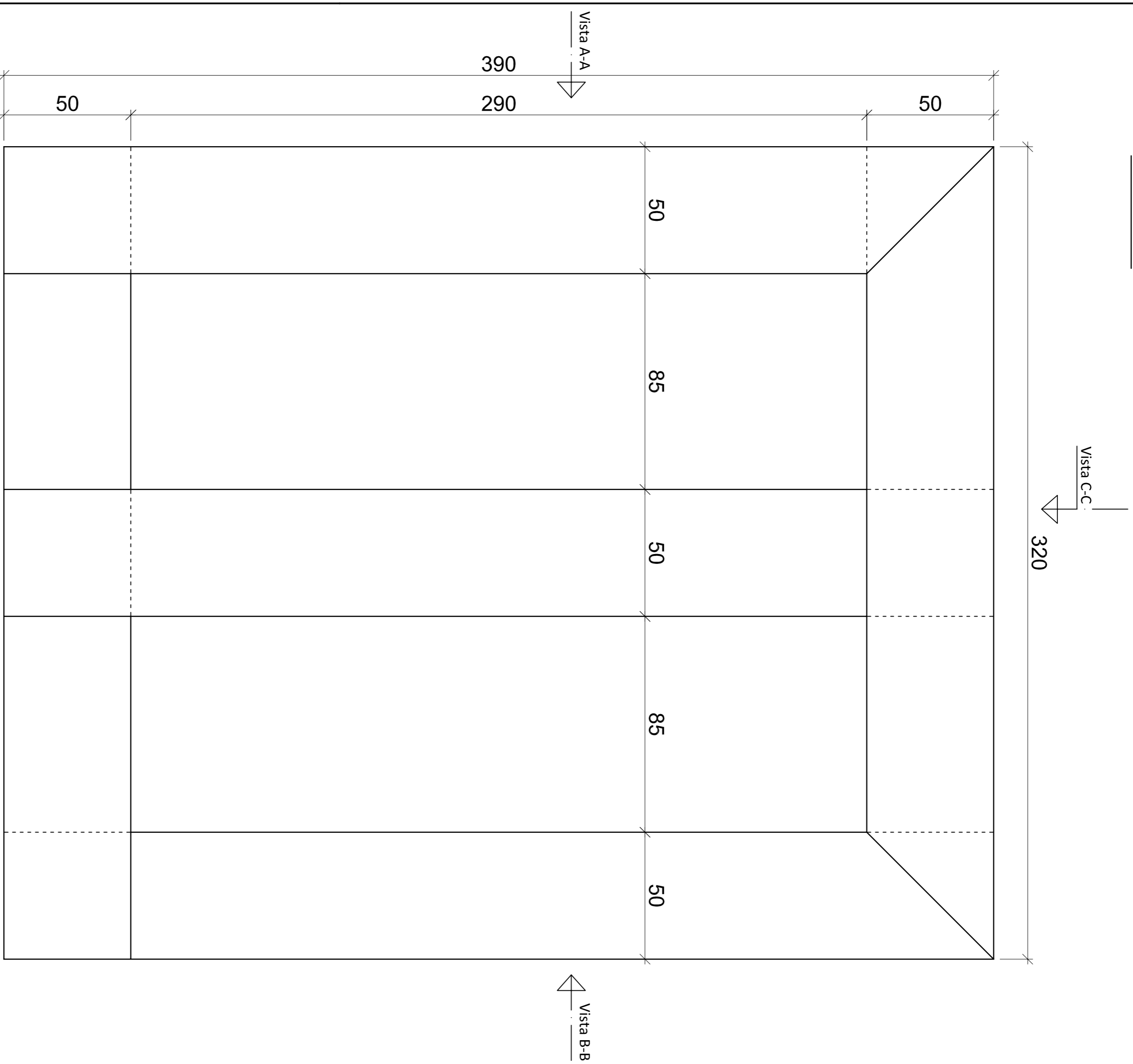
Vista Frontale
